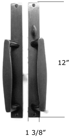
BE671L Escutcheon Patio set shown w/ BP657 Offset El Secreto Grip
