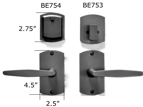
El Secreto BE721-BL155
