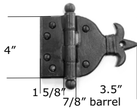
HB369 Full Barrel Fleur de Lis Strap Hinge
