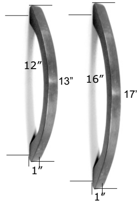
HP773AP-12 HP773AP-16 Arc Pulls (2" projection)
